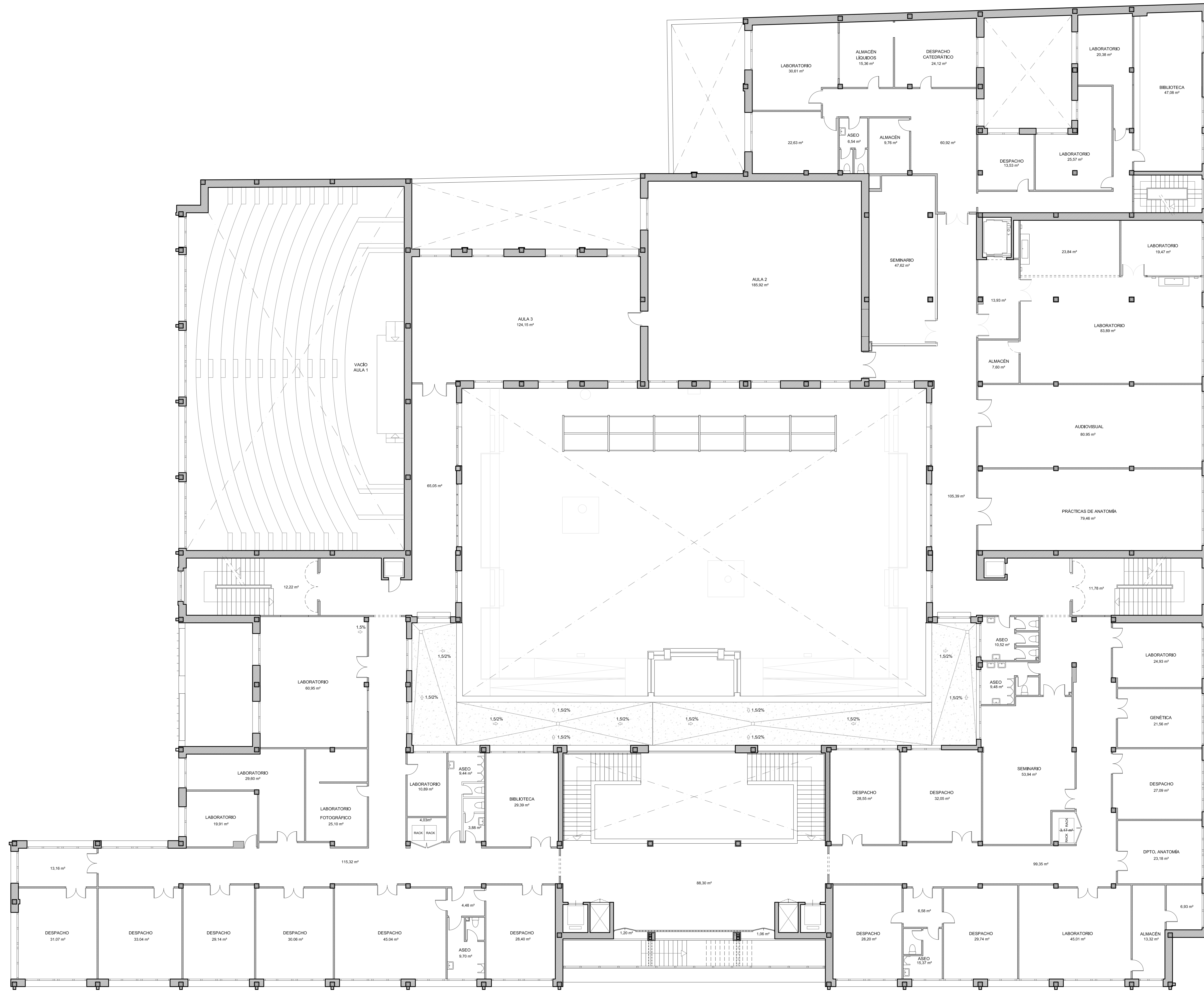
PLANTA PRIMERA
